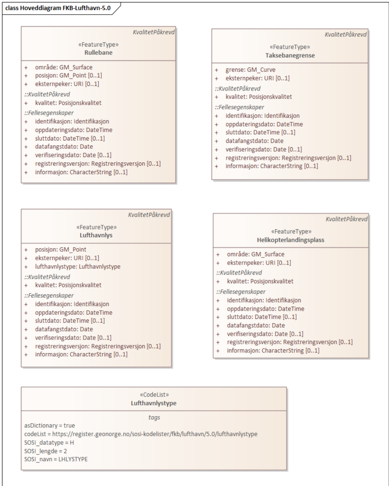
Figur 2. Hoveddiagram FKB-Lufthavn-5.0
